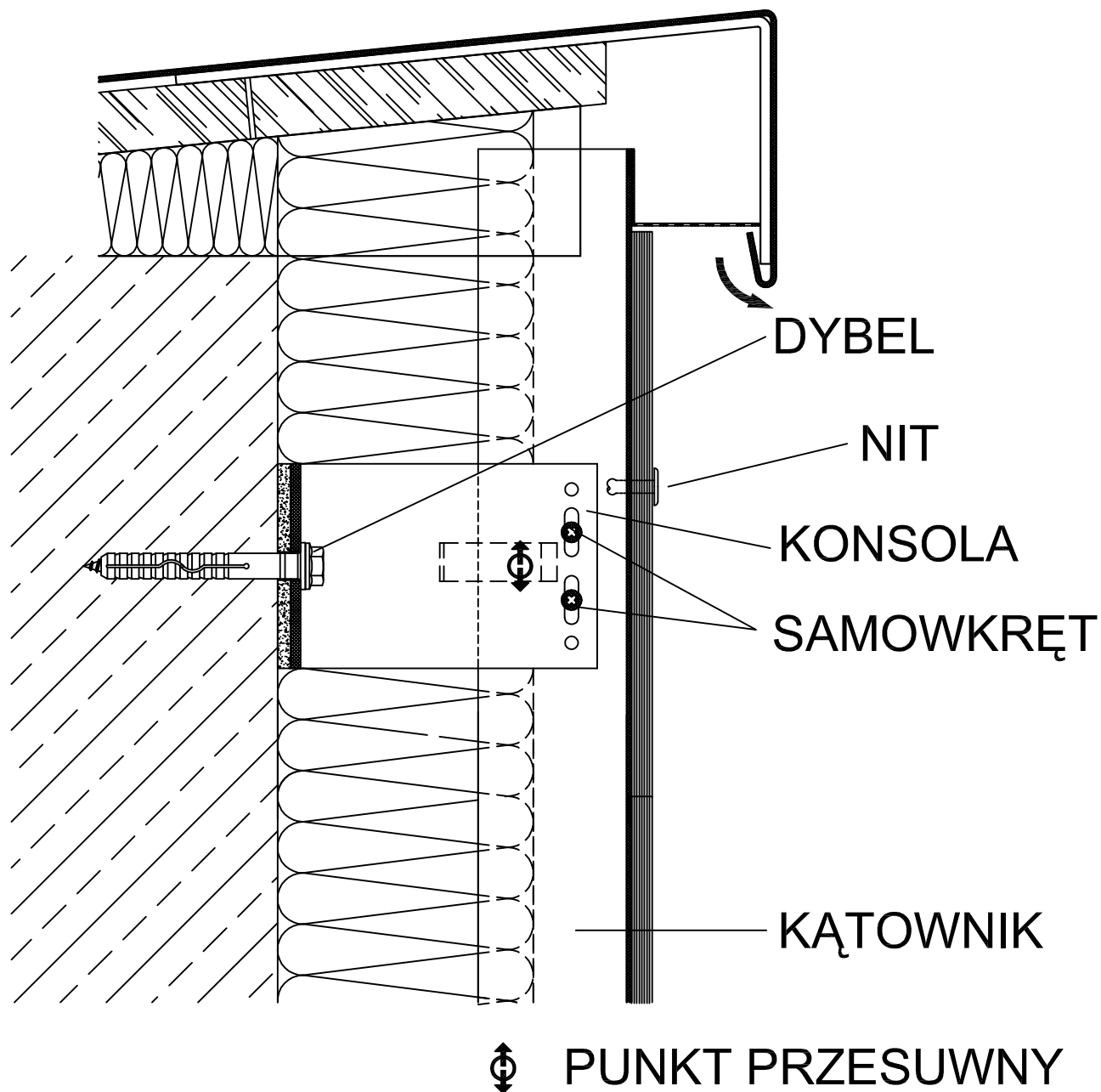
DETAL ATTYKI - PRZEKRÓJ HORYZONTALNY
